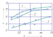
Рис. 1 – Скорость изнашивания деталей
